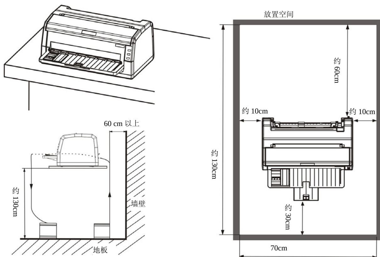
图 2-4 打印机放置
